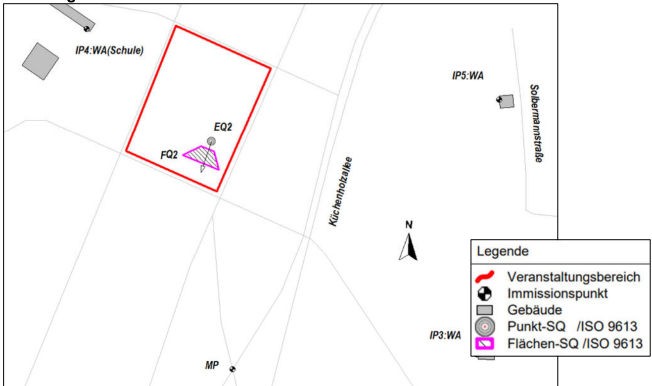
Abbildung: Lageplan Vorzugs-Bühnenstandort EQ2 und Kontroll-Messort MP für Veranstaltungen im Küchenholz
