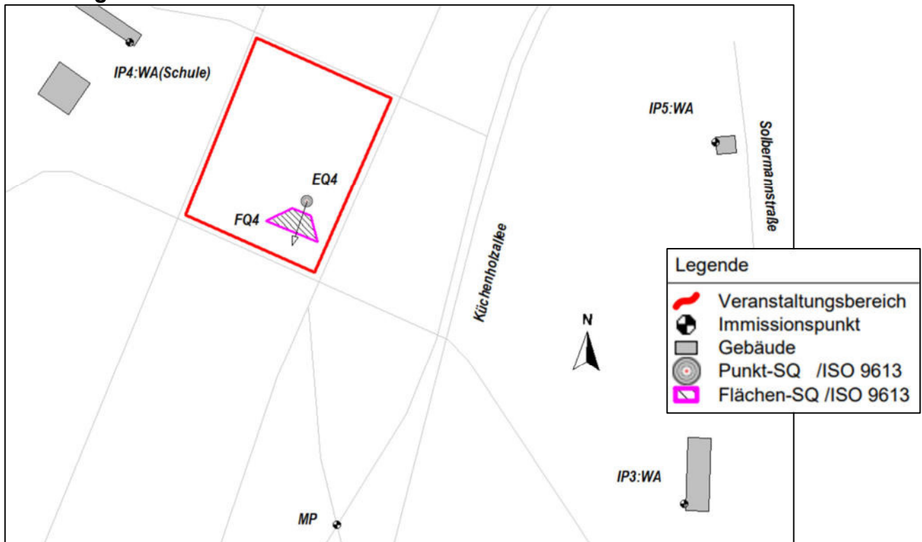
Abbildung: Lageplan Vorzugs-Bühnenstandort EQ4 und Kontroll-Messort MP für Veranstaltungen im Küchenholz
