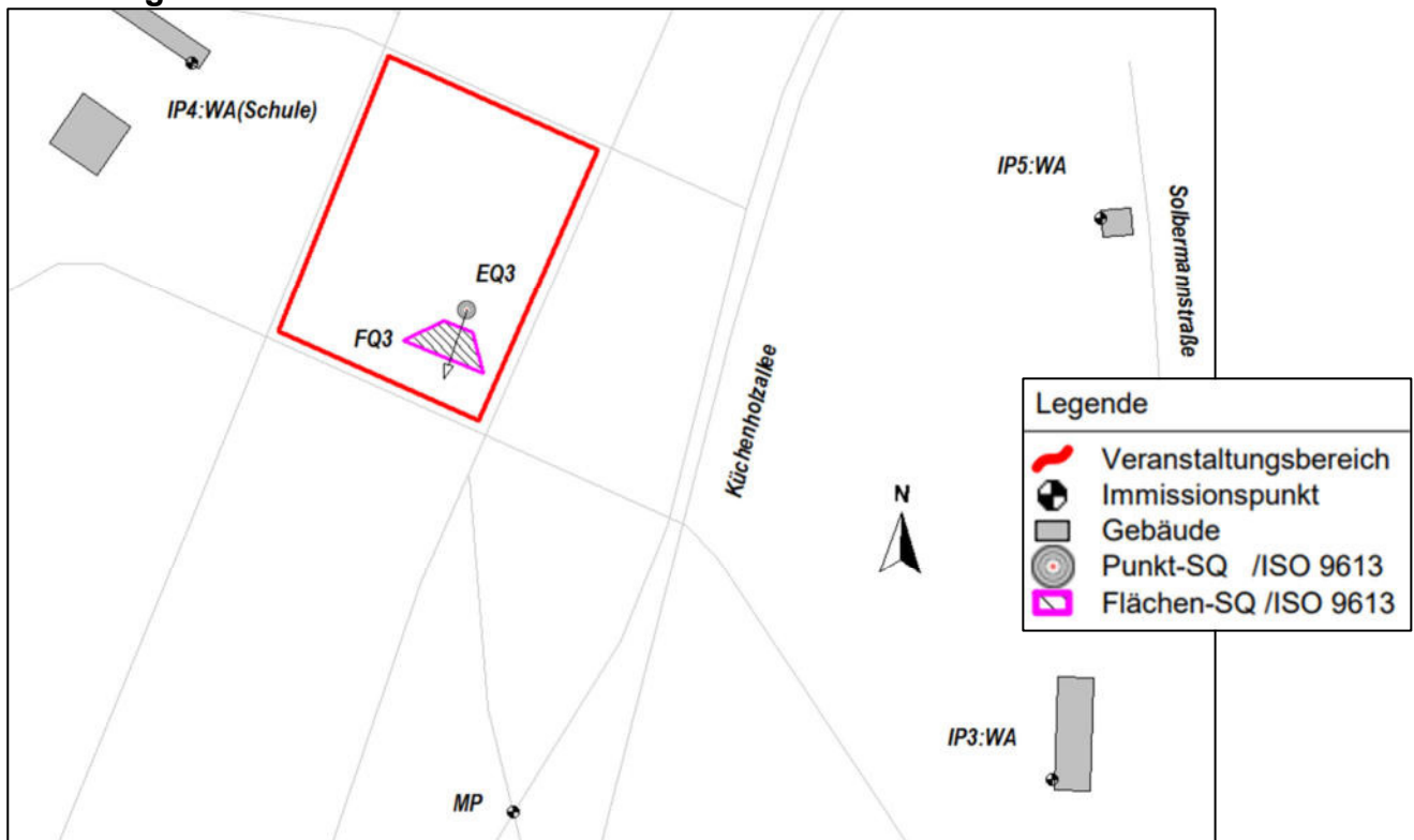
Abbildung: Lageplan Vorzugs-Bühnenstandort EQ3 und Kontroll-Messort MP für Veranstaltungen im Küchenholz
