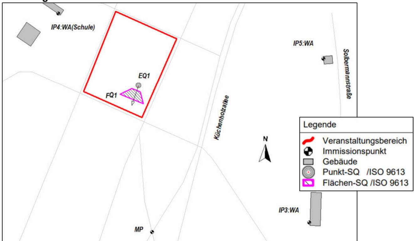
Abbildung: Lageplan Vorzugs-Bühnenstandort EQ1 und Kontroll-Messort MP für Veranstaltungen im Küchenholz
